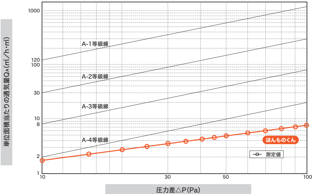
圧力差一単位面積当たりの通気量曲線
